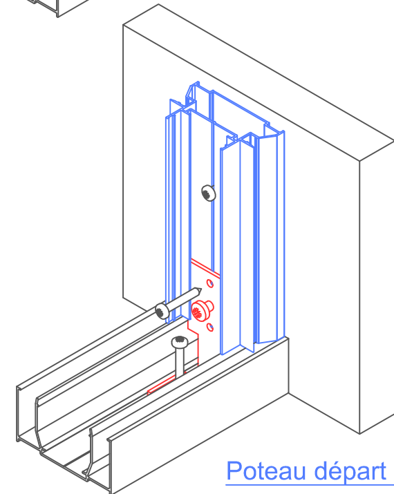
Jonction lisse / Huisserie
