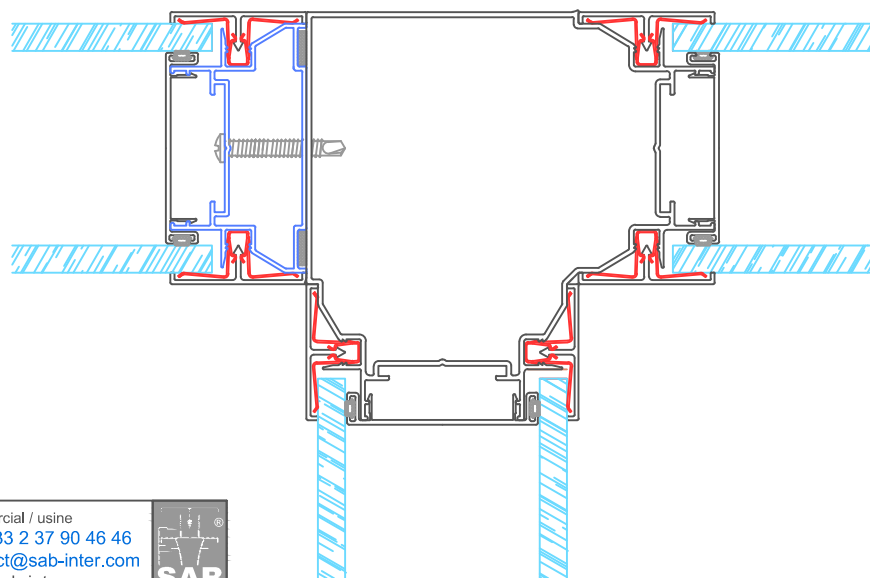
3 départs avec angle droit
