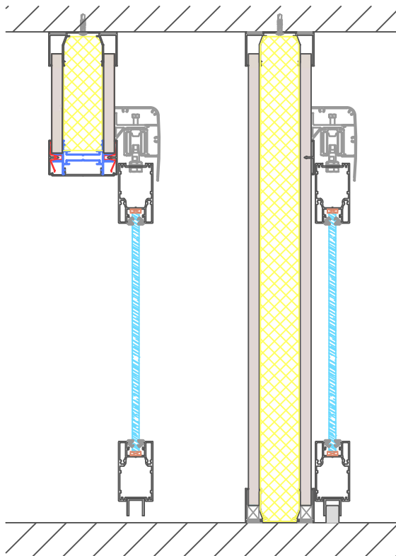
Porte coulissante cadre aluminium avec imposte
