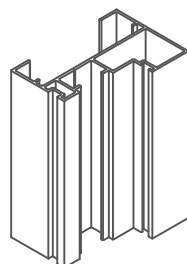
Huisserie ref: EVO400
