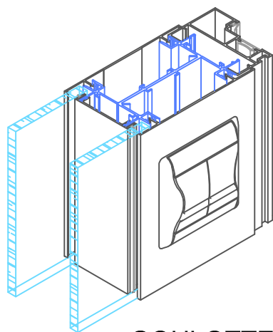
GOULOTTE ELECTRIQUE
