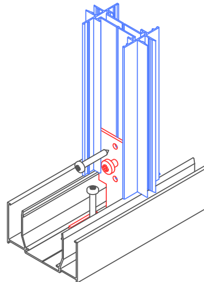
Poteau intermédiaire
