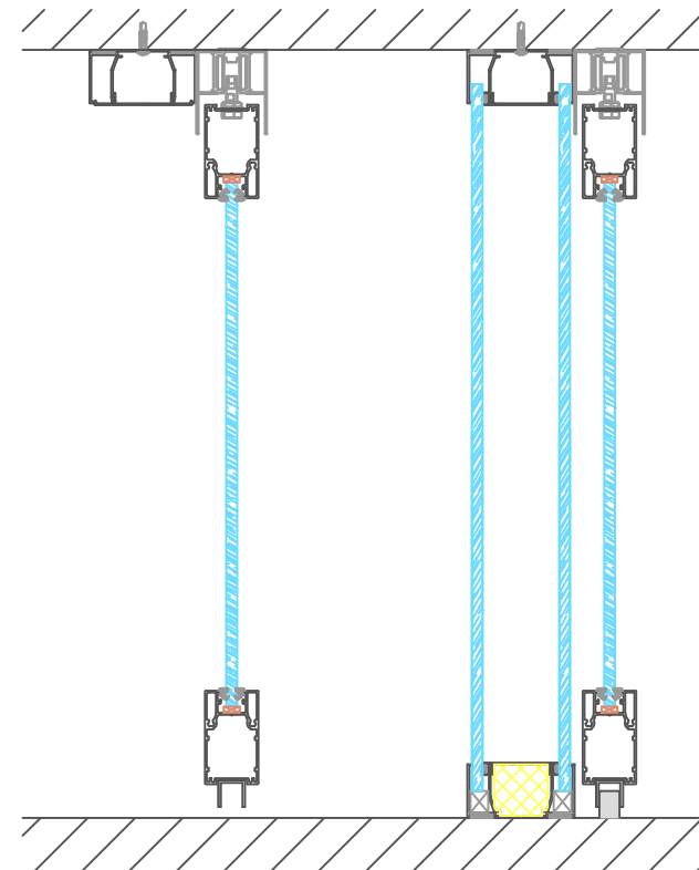
Porte coulissante cadre aluminium toute hauteur
