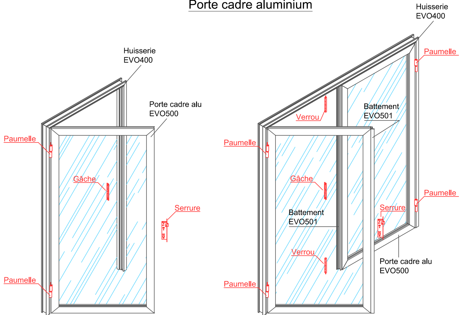
Porte cadre aluminium
