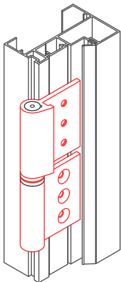
Paumelle réversible en aluminium
