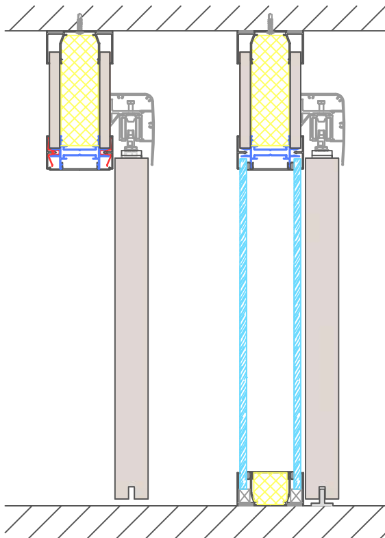
Porte bois coulissante avec imposte
