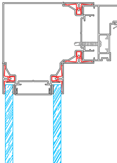
Angle droit
