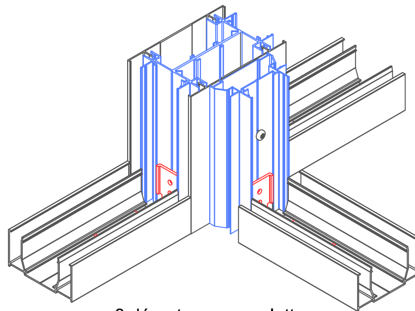
3 départs avec goulotte
